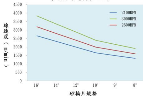
砂輪片線速度(m/min)
