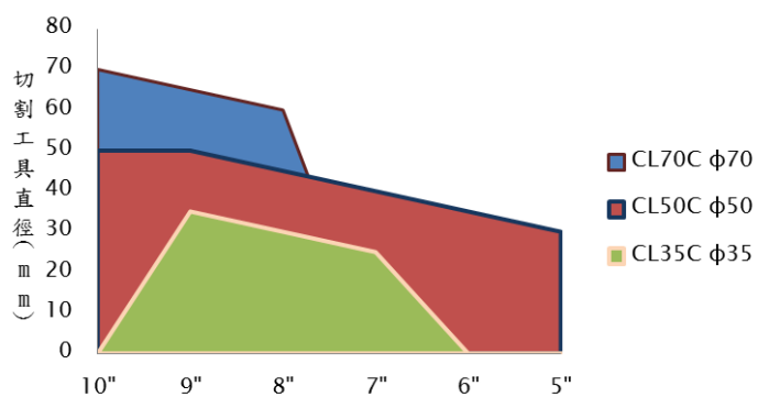
切割範圍示意圖
